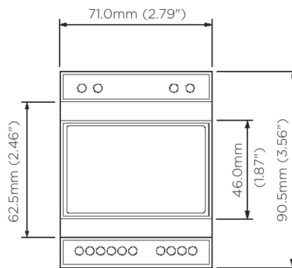
DIN 43880
